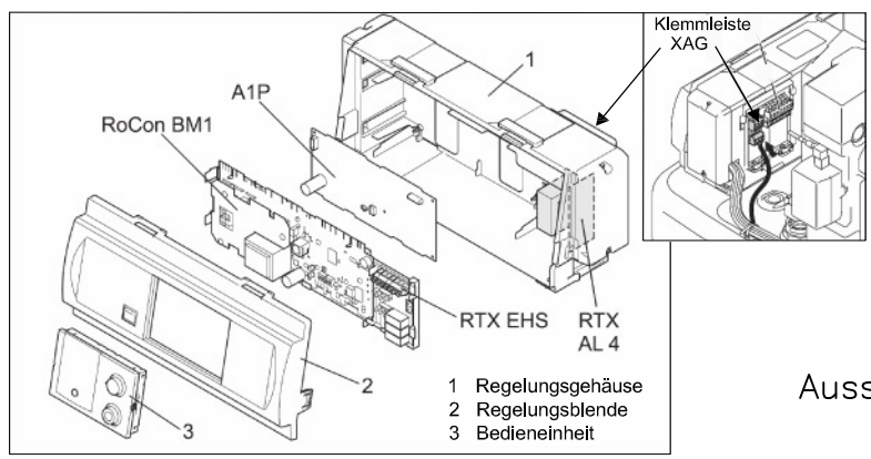
Übersicht Schaltplatten
