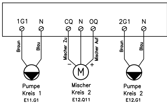
Anschlussklemmen – 3~ Wechselstrom
