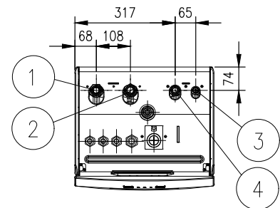
Grundriss
