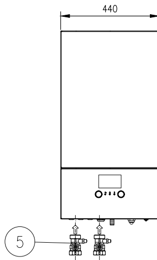
Frontansicht
