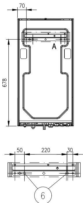
Lochbild
