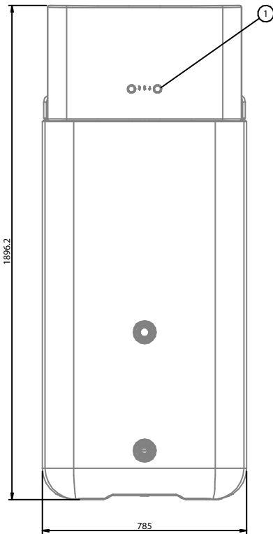
Frontansicht
