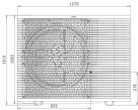
Frontansicht
