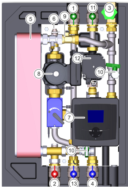
Abb. 1: Frischwasserstation
