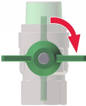
Abb. 28: Hauptabsperrentil geschlossen
