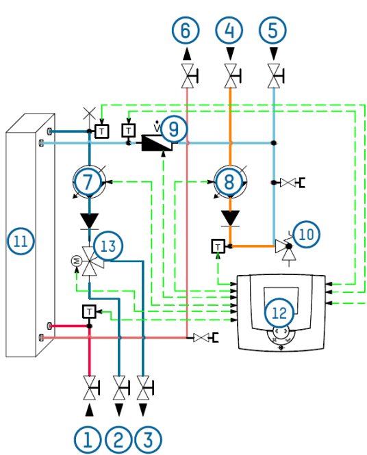
Abb. 36: Hydraulikschema
