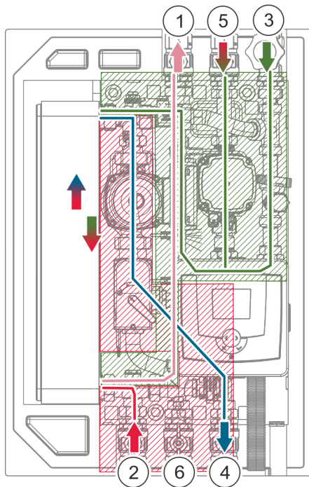
Abb. 6: Übersichtsschema Leitungen
