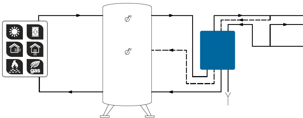
Abb. 35: Anlage-/ Prinzipschema
