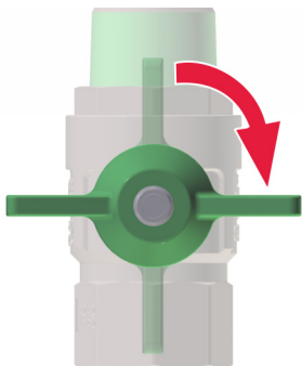
Abb. 33: Hauptabsperrentile schliessen
