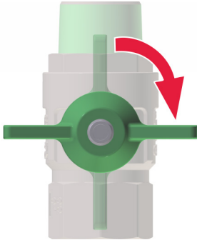
Abb. 25: Hauptabsperrventile schliessen
