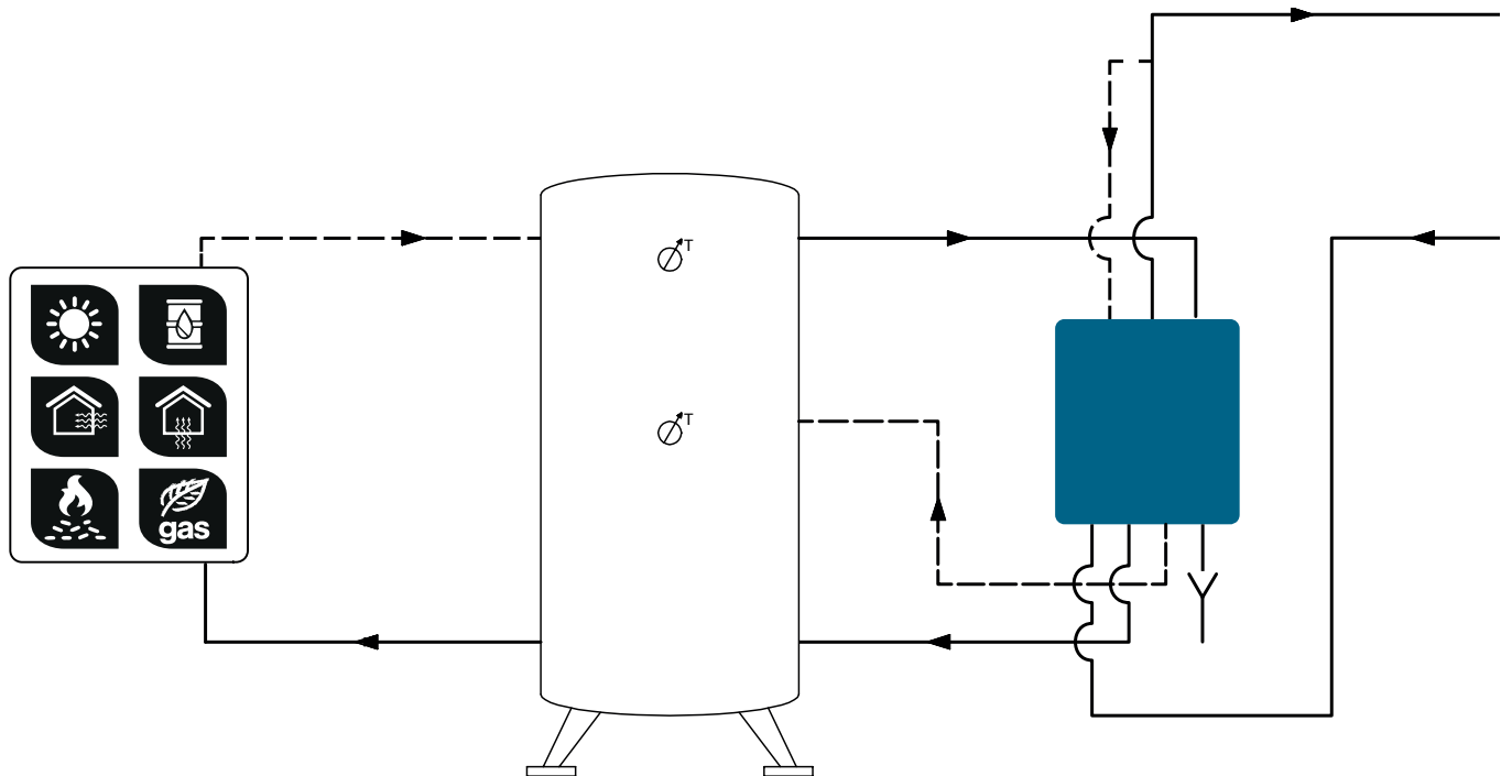
Ill. 10 : Schéma hydraulique CRO 100
