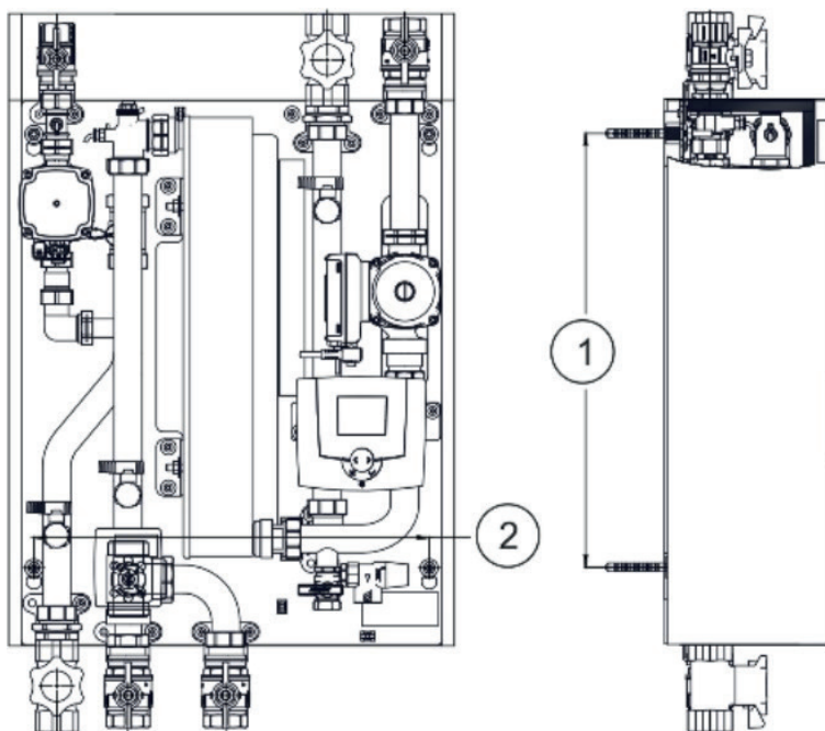
Ill. 20 : Diagramme des trous à percer
