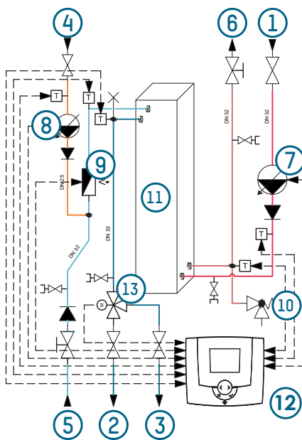
Ill. 10 : Schéma hydraulique CRO 100
