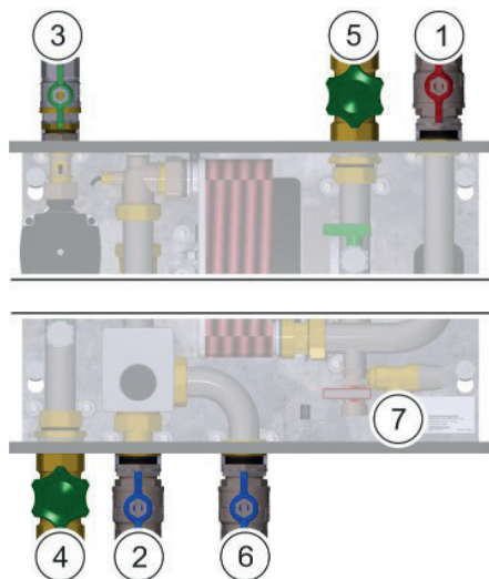
Ill. 22 : Raccordement de la tuyauterie
