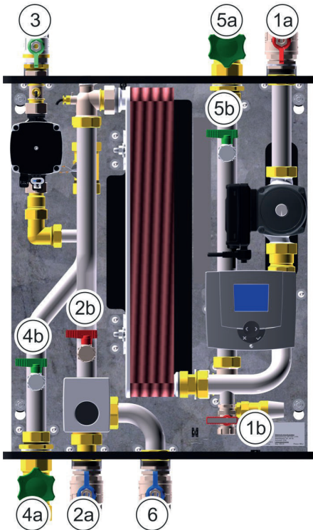
Ill. 26 : Groupe de charge
