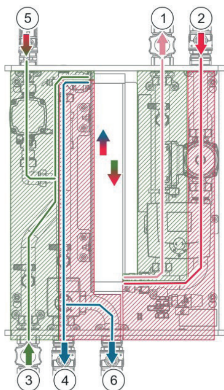
Ill. 6 : Schéma d'ensemble des conduites
