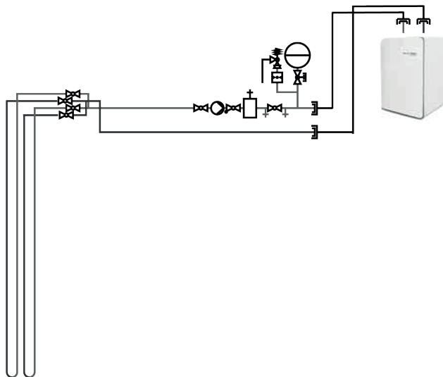
III. 14 Schéma hydraulique du circuit primaire (sonde géothermique à saumure)
