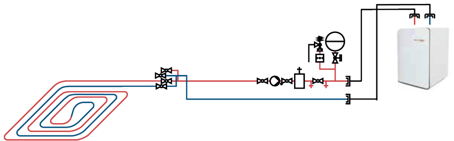
Ill. 14 Schéma hydraulique du circuit primaire (capteur souterrain horizontal)
