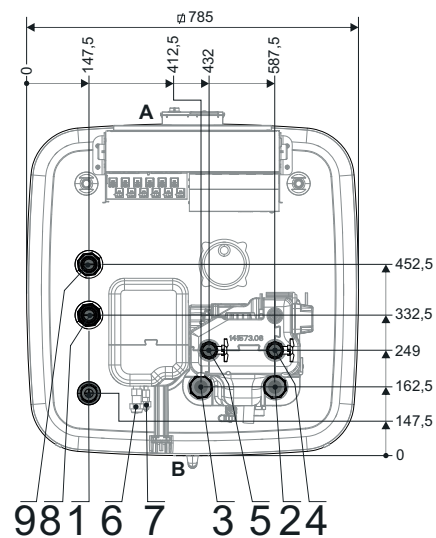
Proiezione orizzontale
