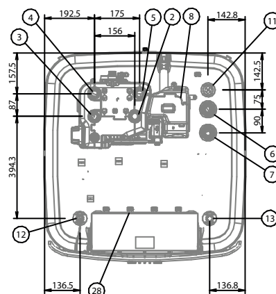
Proiezione orizzontale
