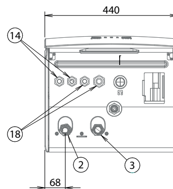
Proiezione orizzontale
