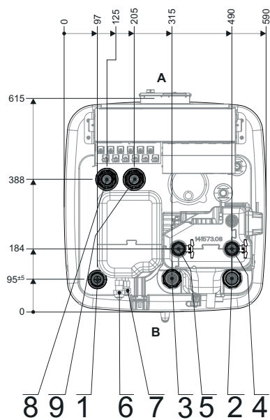
Proiezione orizzontale
