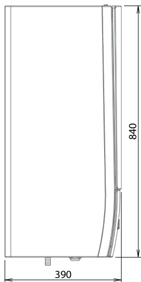
Veduta laterale
