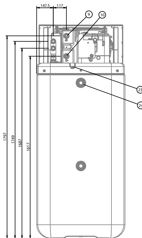
Vista posteriore
