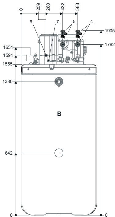
Veduta frontale
