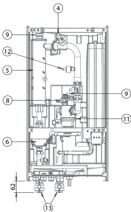
Veduta frontale
