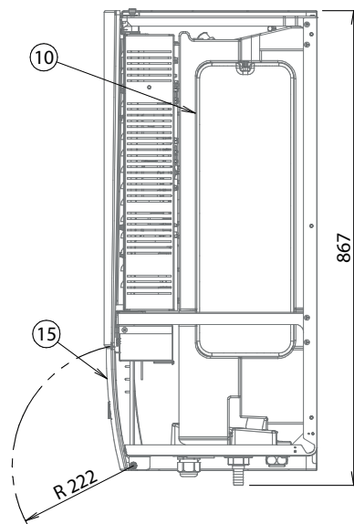
Veduta laterale
