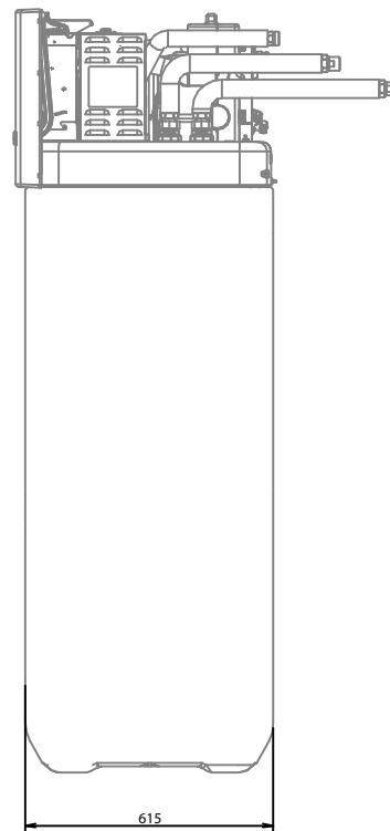
Veduta laterale
