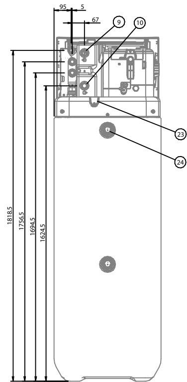
Vista posteriore
