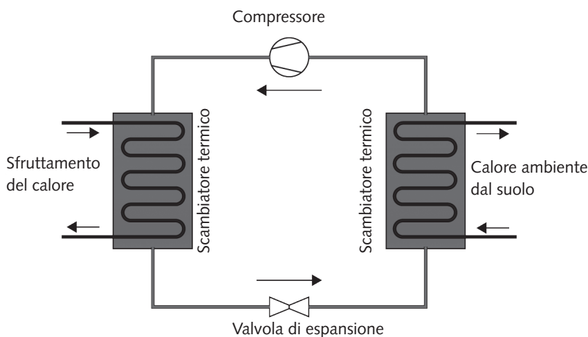
Abb. 1 Principio di funzionamento della pompa di calore
