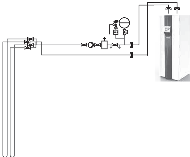
Fig. 9 Schema idraulico circuito primario (sonda salamoia)
