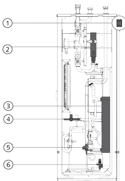
Fig. 2 Pompa di calore vista frontale
