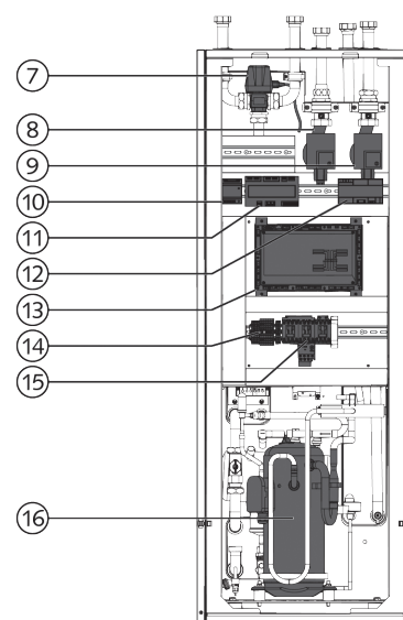
Fig. 3 Pompa di calore vista frontale aperta
