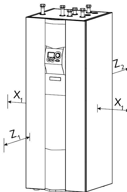
Fig. 7 Distanze minime consigliate
