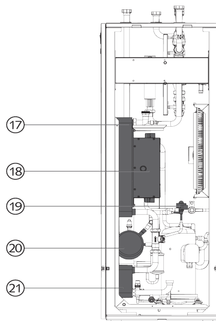
Fig. 4 Pompa di calore vista laterale aperta
