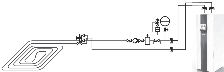
Fig. 8 Schema idraulico circuito primario (collettore geotermico)
