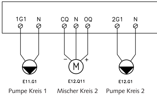
Anschlussklemmen – 3-Wechselstrom
