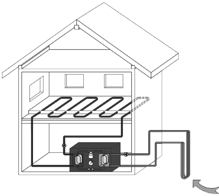
Domotec Sole-Wasser-Wärmepumpe mit Erdsonde
