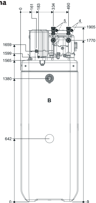
Veduta frontale
