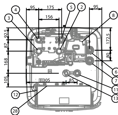
Proiezione orizzontale
