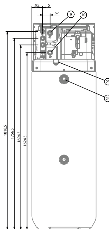
Vista posteriore
