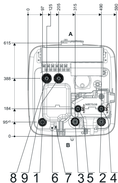
Proiezione orizzontale
