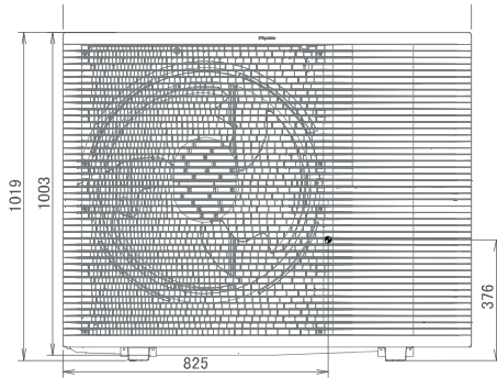
Veduta frontale
