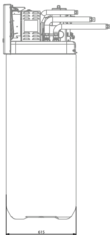
Veduta laterale
