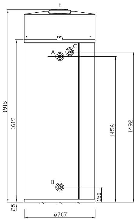
Seitenansicht
