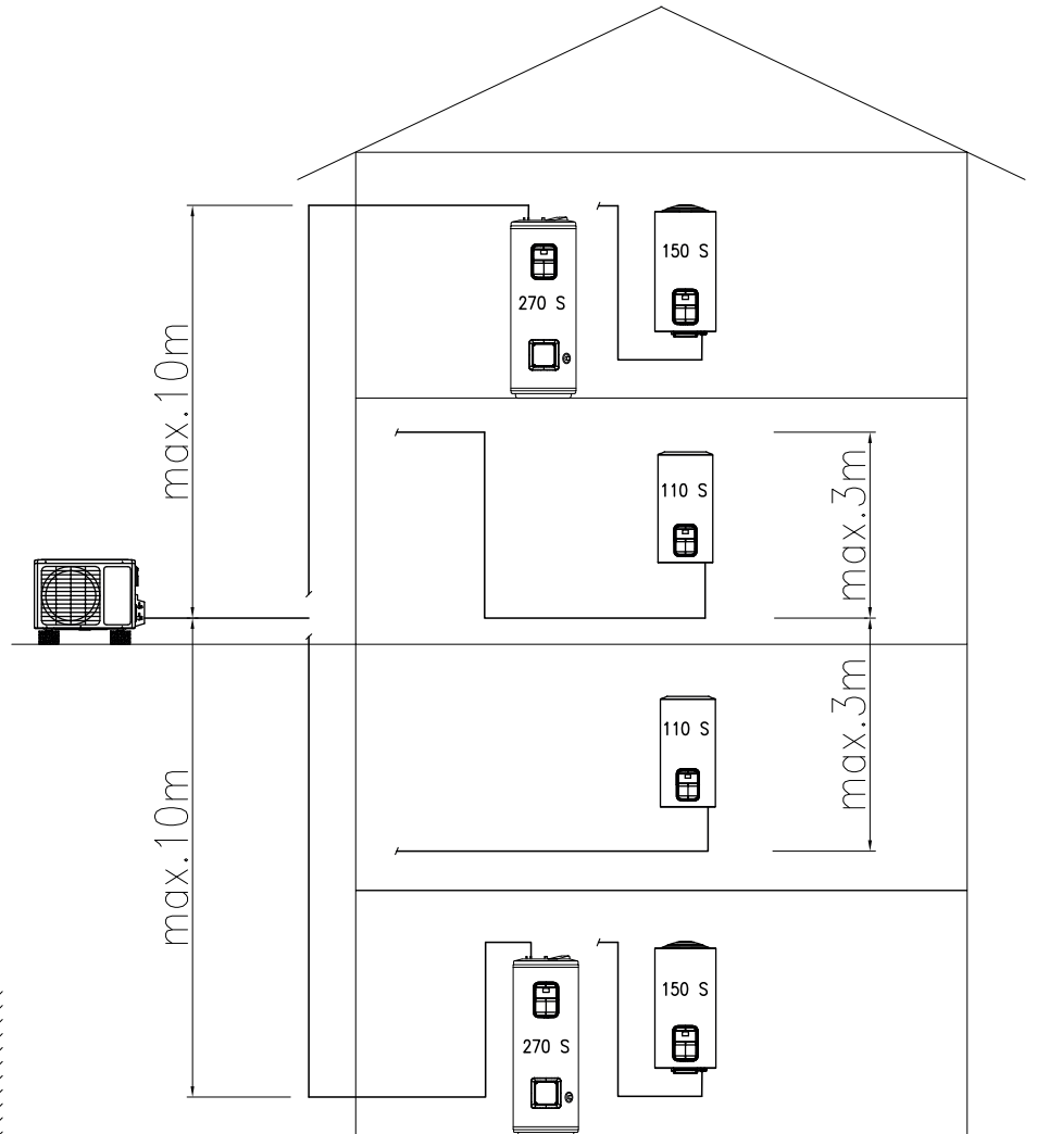
Maximaler Höhenunterschied
