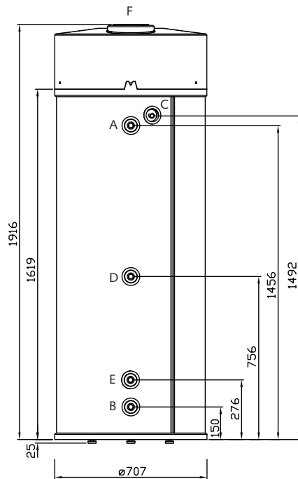
Seitenansicht
