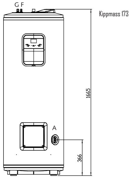
Frontansicht
