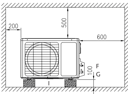
Minimale Wandabstände
