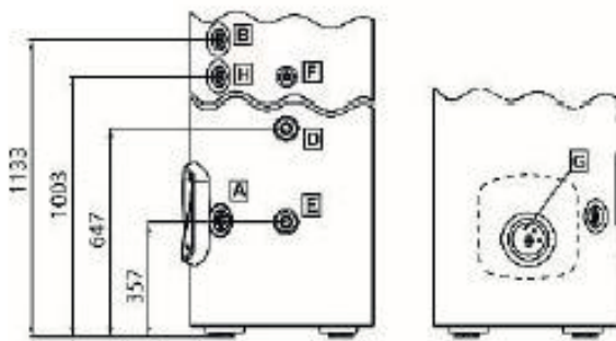
Anschlüsse NUOS P 240 W1
