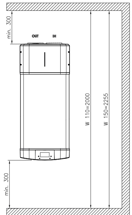
Distance minimum du mur
