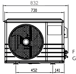
Vue de face unité extérieure
