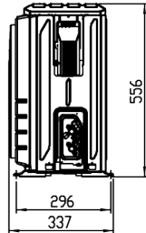
Vue latérale unité extérieure
