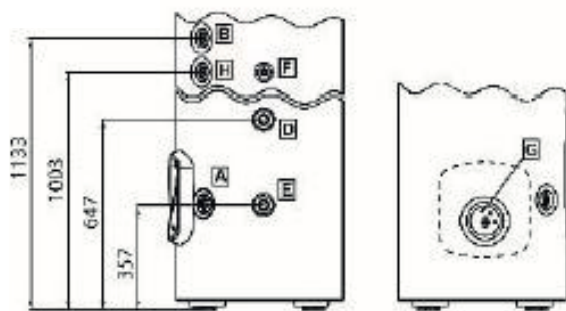
Raccordements NUOS P S 240 W1
