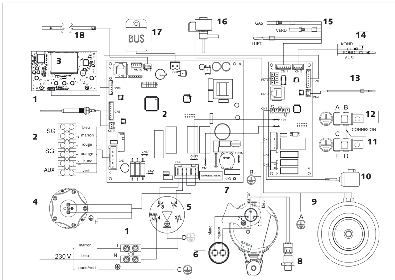
III. : Schéma électrique
