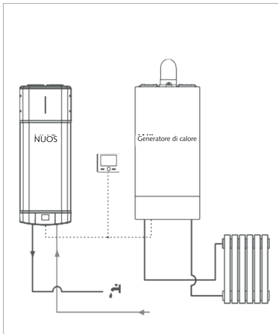
Fig.: Tipi di impianto (A)
