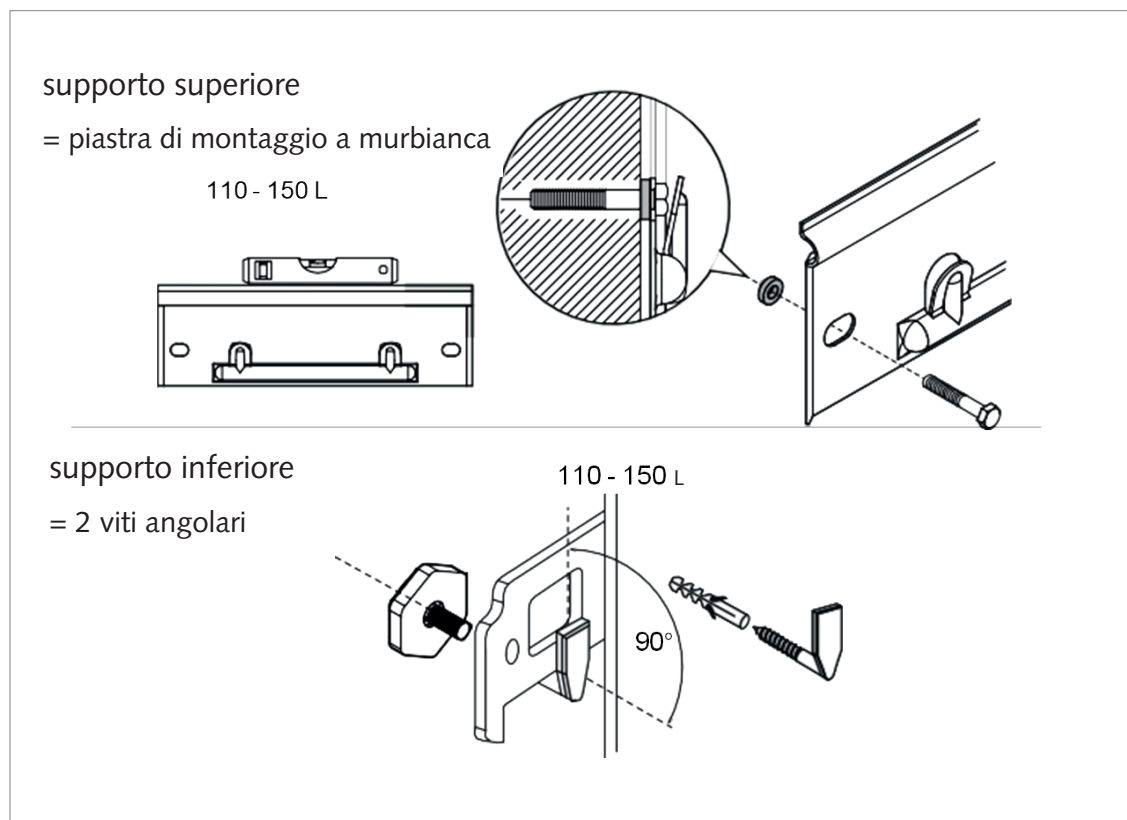
Fig.: Montaggio a parete
