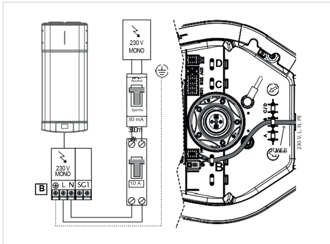
Fig.: Collegamento elettrico permanentess
