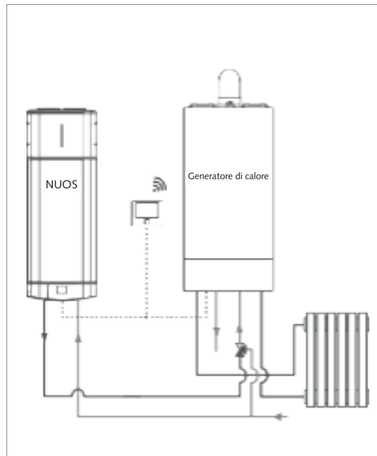
Fig.: Tipi di impianto (B)
