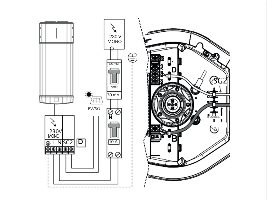
Ill. : PV ou SMART GRID (SG2)
