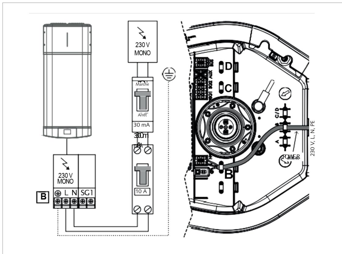
Ill. : Raccordement électrique permanent
