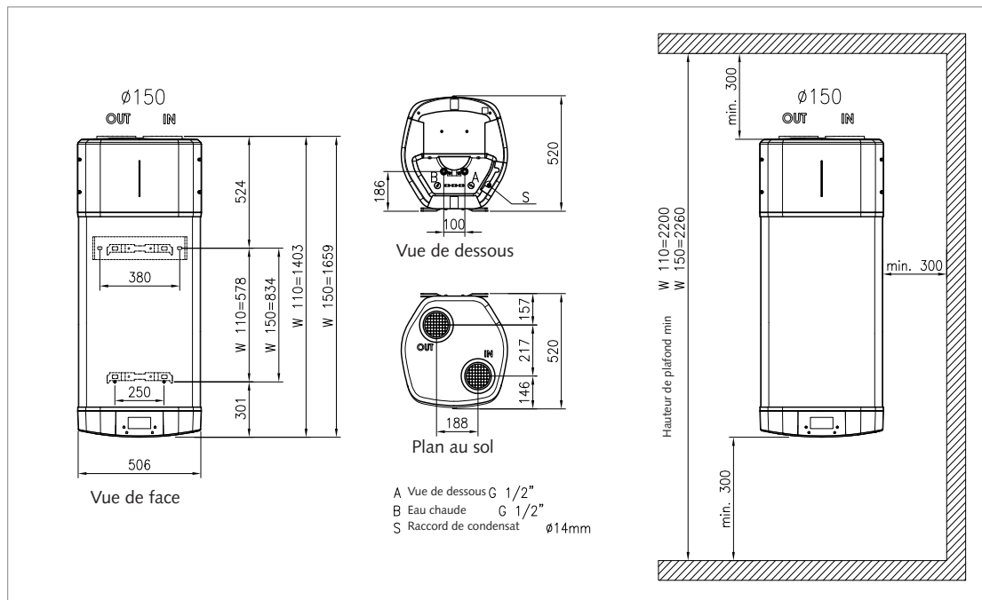
III. : Dimensions
