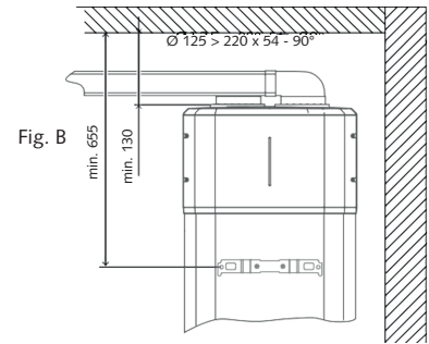
Ø 125 CANALISATION, AVEC ADAPTEUR
