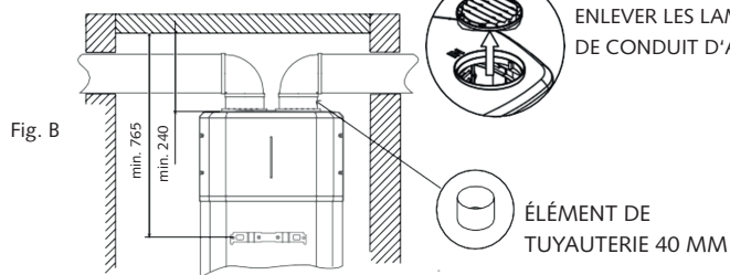
CANALISATION, Ø 150 PAS D'ADAPTEUR
