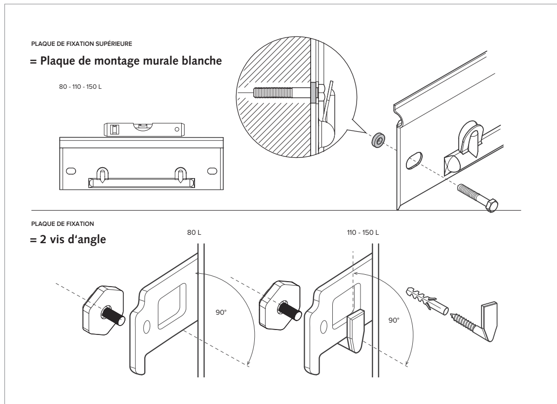
Ill. : Montage mural
