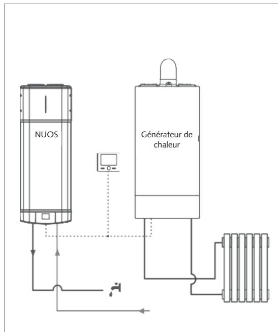
Ill. : Types d'installations (A)
