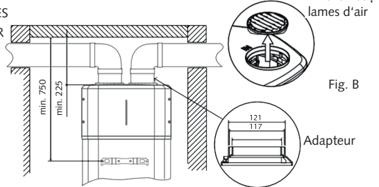
Ø 125 CANALISATION, AVEC ADAPTEUR
