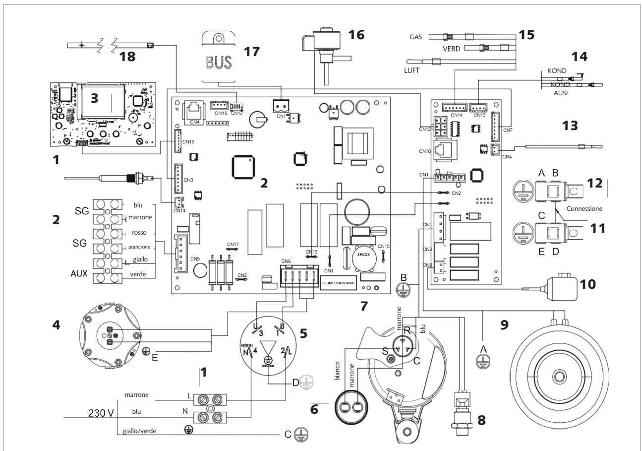
Fig.: Schema elettrico
