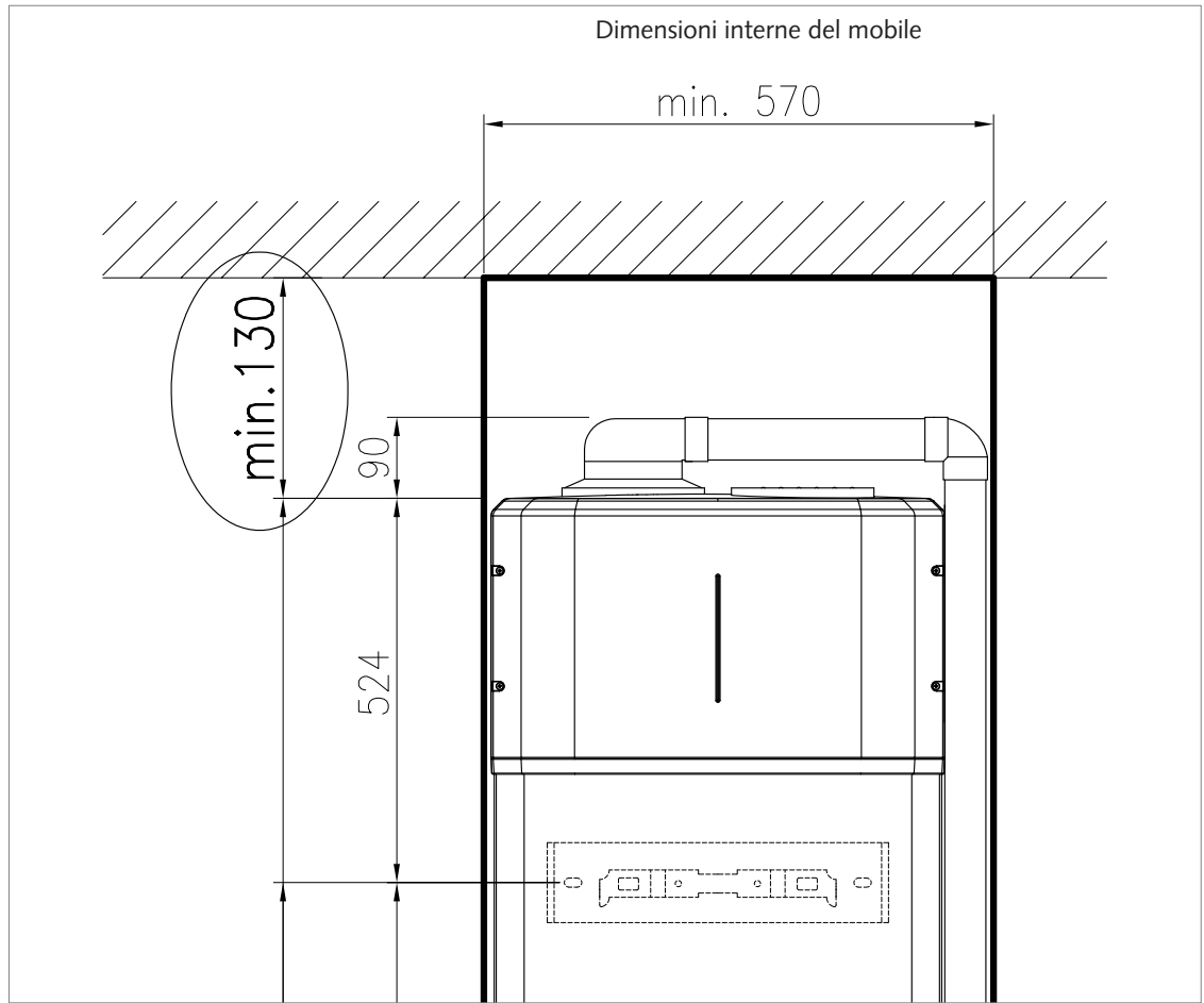
Fig.: Distanza minima dal soffitto
