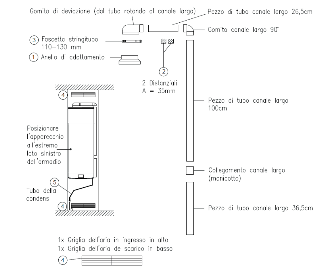
Fig.: Istruzioni per l'installazione del condotto dell'aria di scarico
