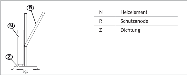
Abb. 3: Heizelement
