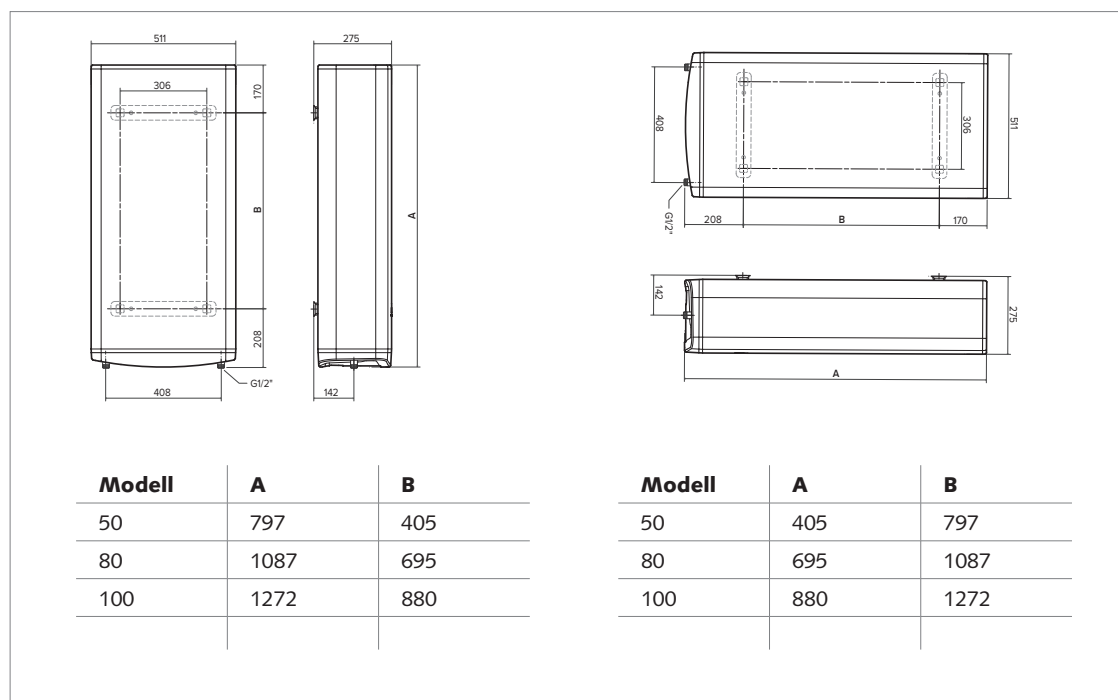
Abb.: Technische Daten WF 050 - WF 100 E / WFHL 050 E - WFHL 100 E
